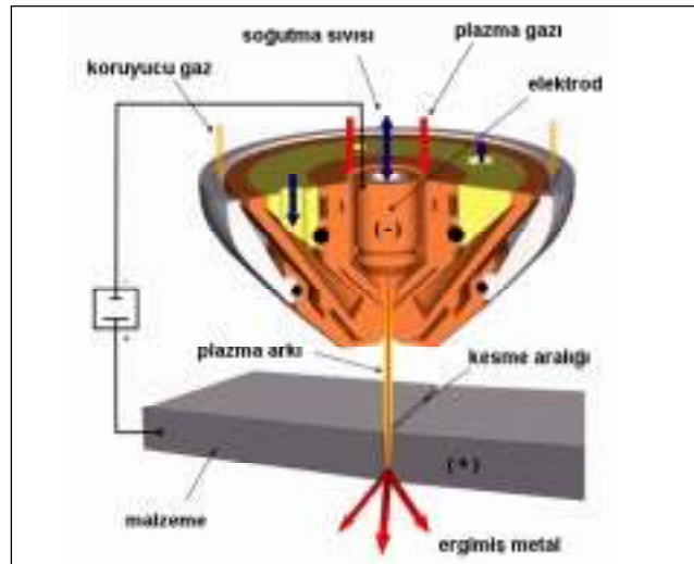
Şekil 1. Plazma ile Kesme
