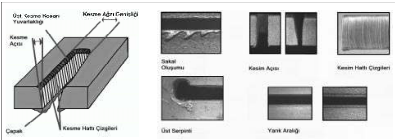
Şekil 8. Plazma Kesmede Kaliteyi Belirleyen Etmenler
