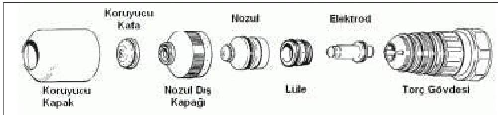
Şekil 4. Torç Kafası Parçaları (Kaynak: Hypertherm)
